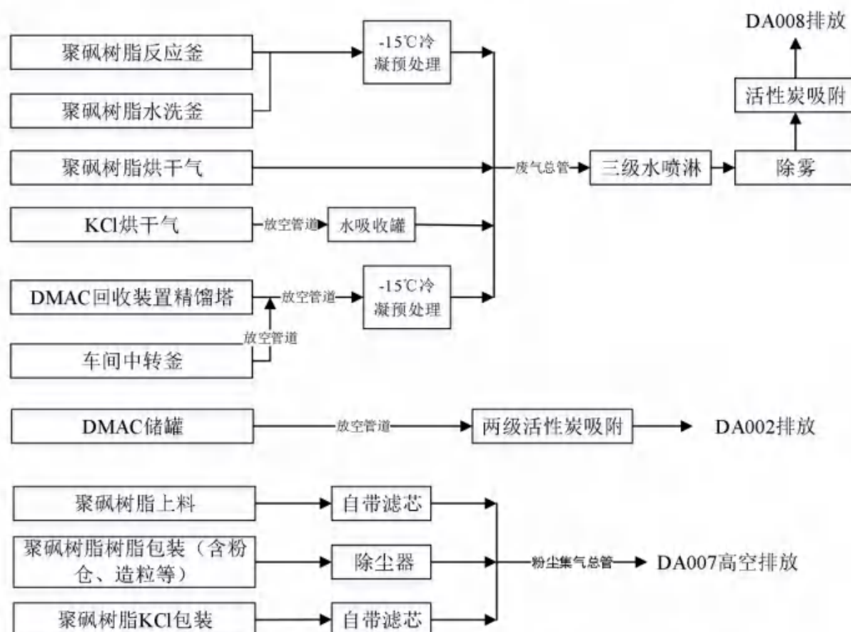
图 4.1-6 本次先行建设内容废气处理设施流程简图
