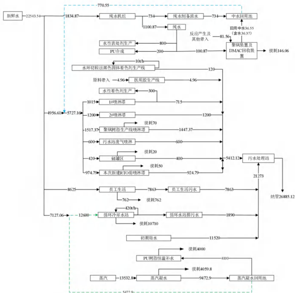
图 3.4-2 先行建设内容实施后全厂满负荷运行时水平衡 (根据调试数据折算) (单位: t/a)
