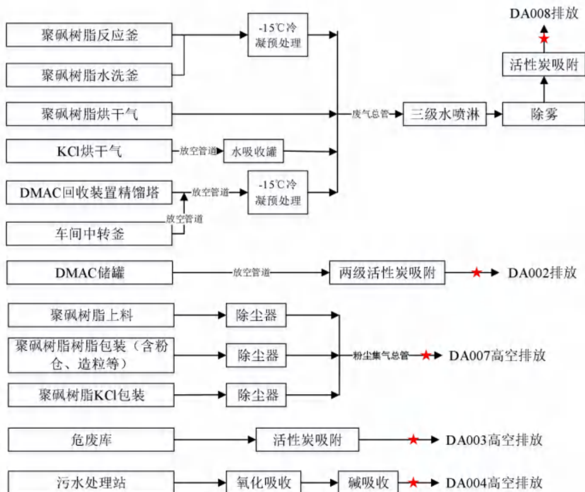
图 7.1-1 本项目废气有组织监测点位图
