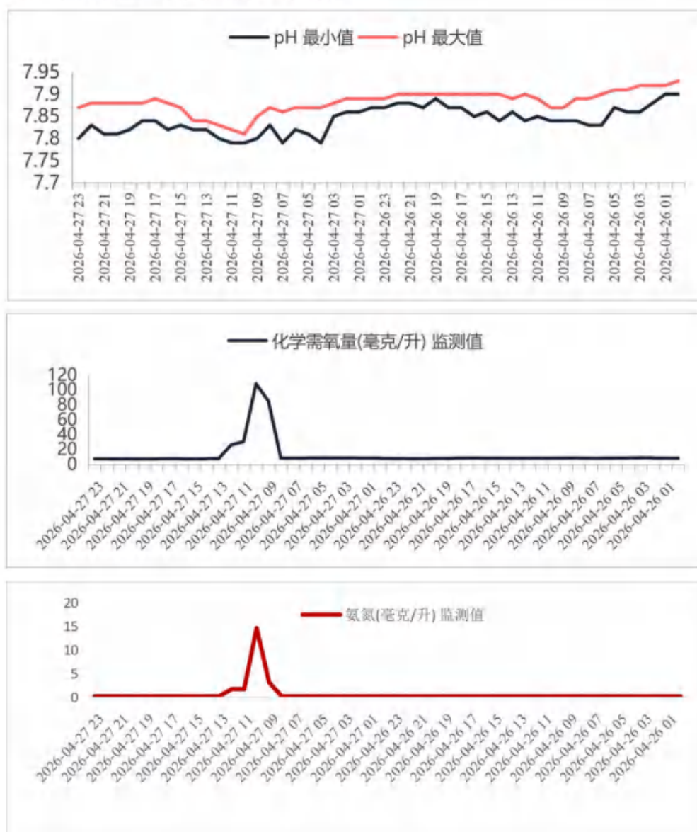
图 9.2.1-1 废水总排口在线监测结果图
