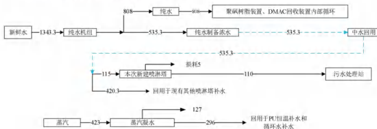
图 3.4-1 本次先行建设内容水平衡图（单位：t/a）
